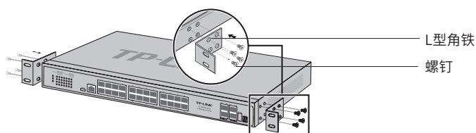
图2-2 角铁安装示意图
