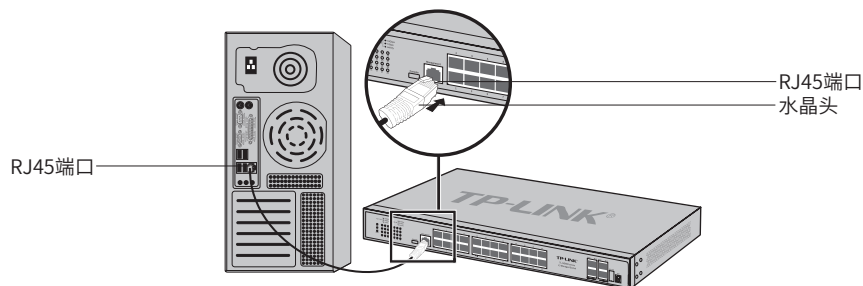
图3-1 RJ45端口连接示意图
