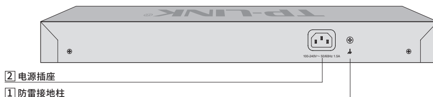
图1-4 后面板示意图
