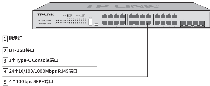
图1-3 TL-NS650-24G4T前面板示意图
