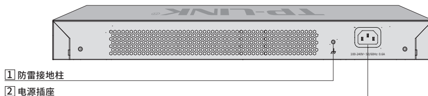
图1-5 后面板示意图
