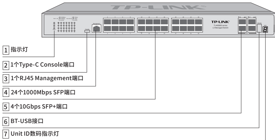
图1-1 TL-NS660-24F4T前面板示意图
