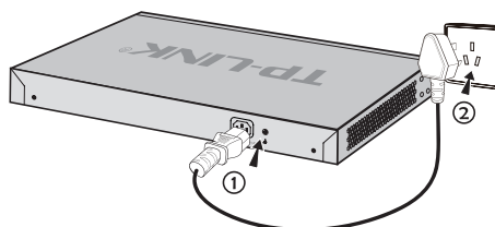
图3-4 电源线连接示意图
