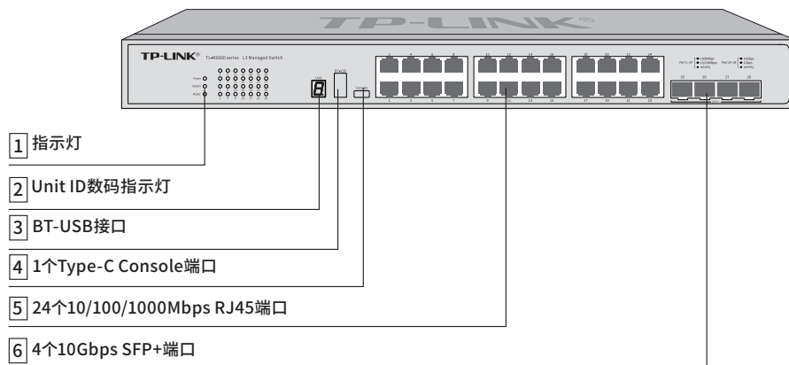
图1-2 TL-NS660-24G4T前面板示意图
